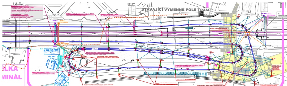
Navržené řešení trolejového vedení v oblasti terminálu Nádraží Veleslavín. Zdroj: Projektová dokumentace Pragoprojektu
