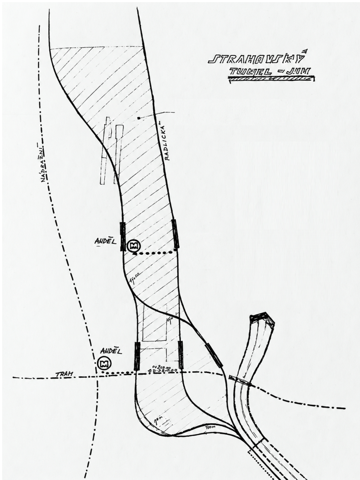
Náčrtek možného vedení nekonvenčního metra do Strahovského tunelu (ve spodní části) ukazuje komplikované zaústění do východní tunelové trouby s oblouky o malých poloměrech. (zdroj: archiv DPP)
