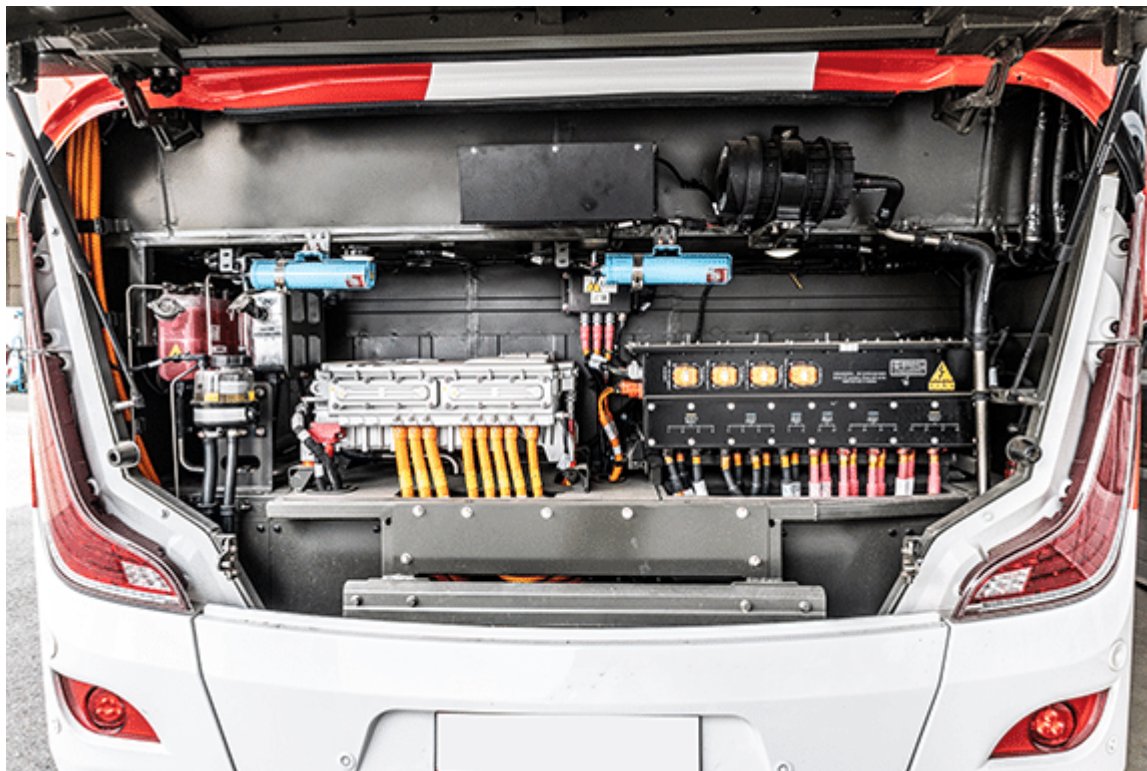
Pohled do zadní části vozidla s elektroinstalací a bateriemi. (zdroj: Blaguss)
